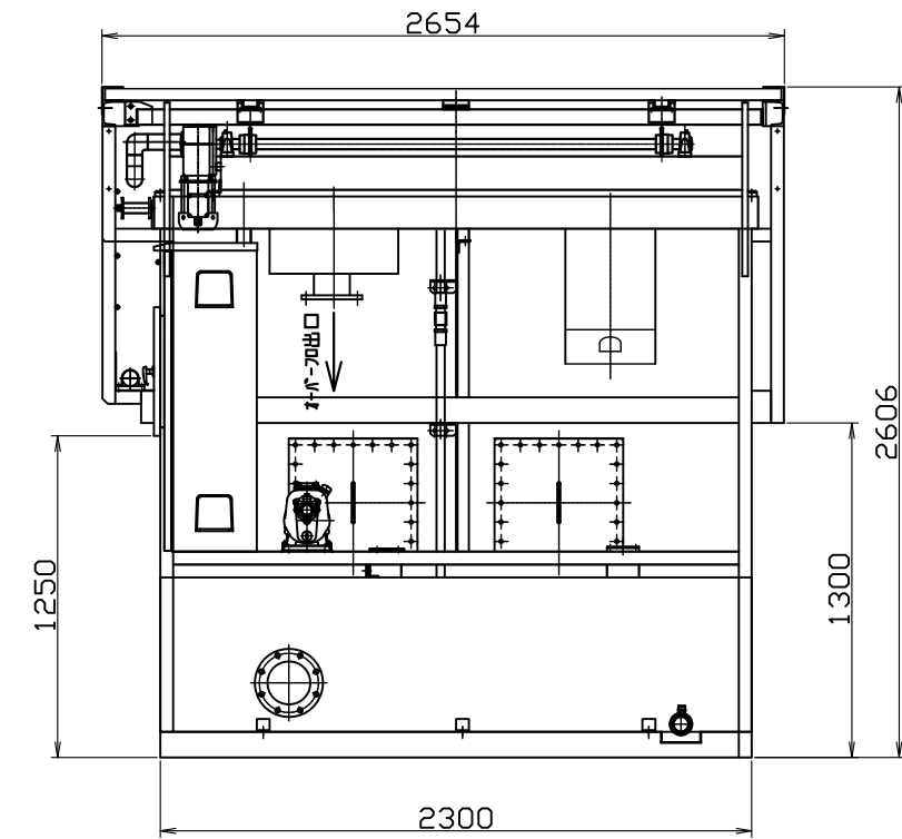
A矢視
