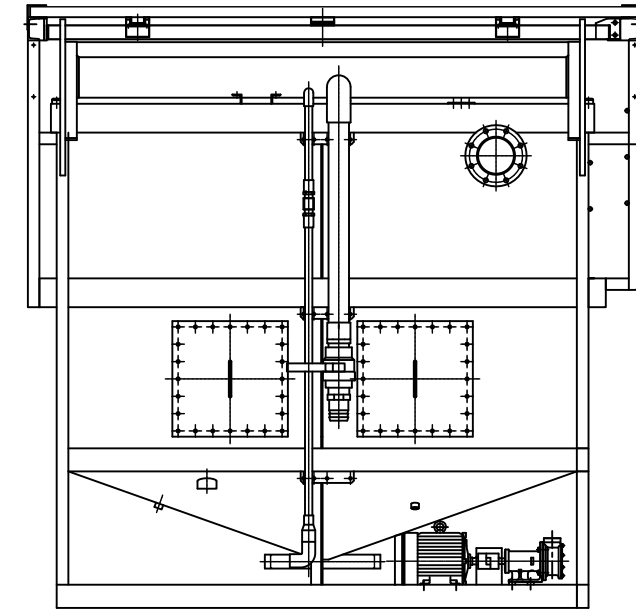
A矢視
